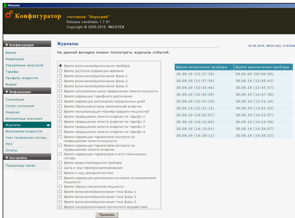
Рисунок 6.9 – Вкладка «Журналы»
