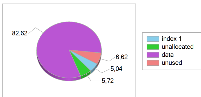
Место, занятое файлами данных (%)
