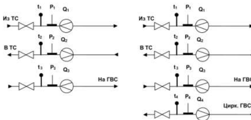
а) Открытая двухтрубная система отопления + тупиковая ГВС
