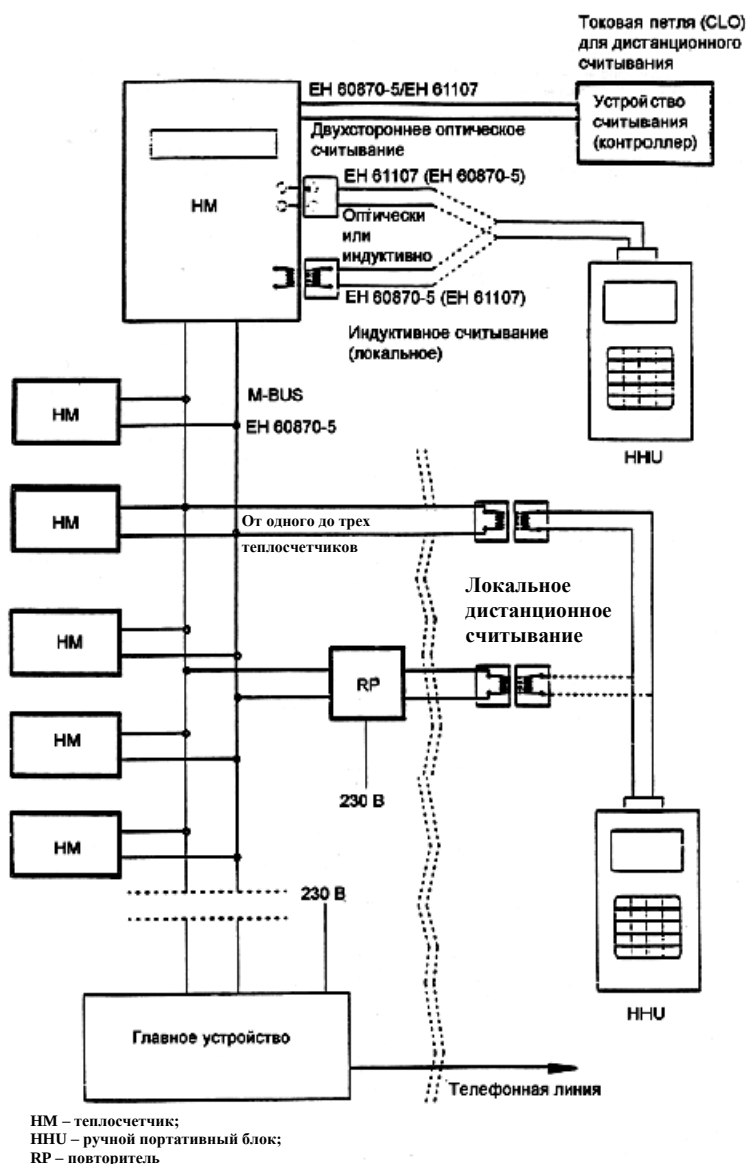
Рисунок 1 – Интерфейсы связи теплосчетчиков
