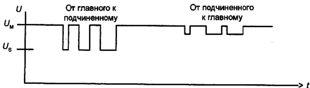
Рисунок В.1 – Зависимость напряжения от времени
