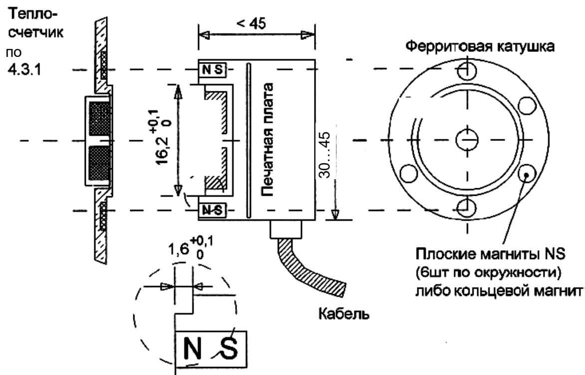
Рисунок D.1 – Расположение компонентов и размеры
