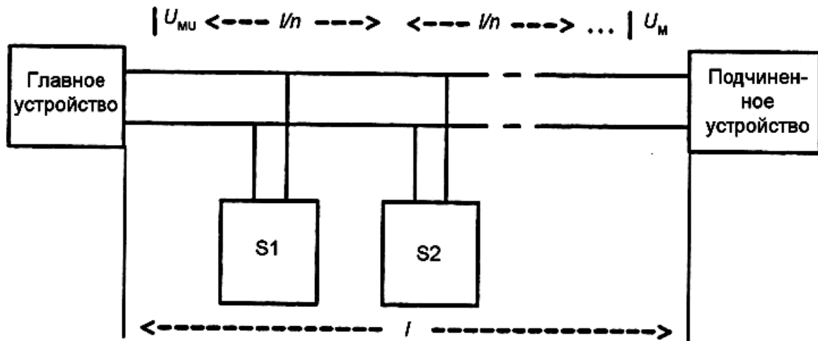
Рисунок В.3 – Тестовое оборудование для М-Bus ( l )
