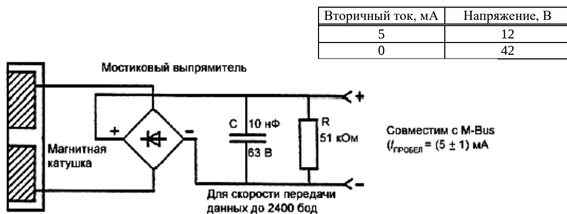
Рисунок 4 – Электрические элементы в теплосчетчике
