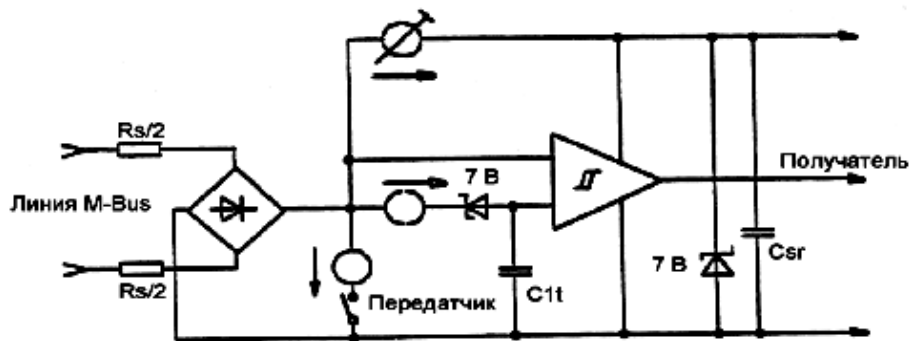
Рисунок 2 – Схема для интерфейса М-Bus
