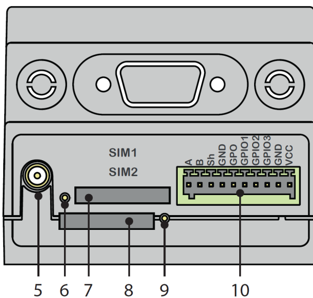
Рис. 2.3 Вид сзади
