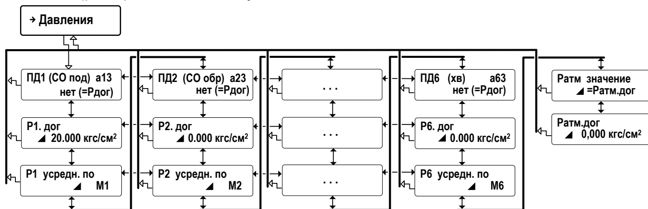
Рис.5. Структура подменю «Давления».
